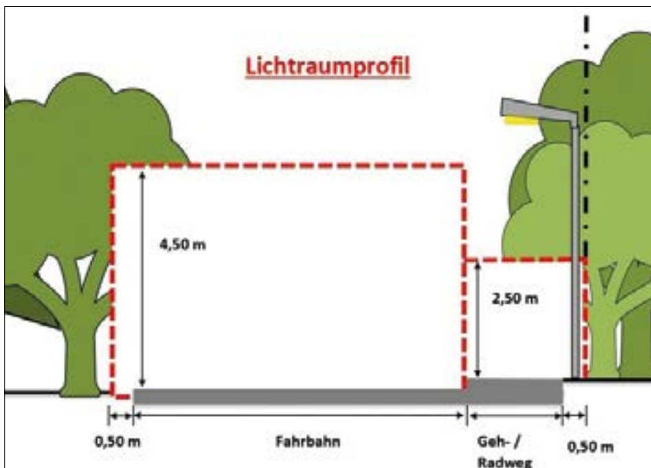
Lichtraumprofil Strasse.
