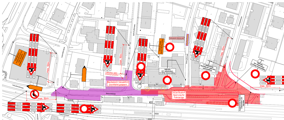
Ausschnitt Signalisationsplan Etappe 2 vom 15. Dezember 2024 bis Anfangs 2026
